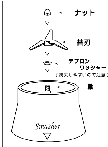
ミキサー部構成図
