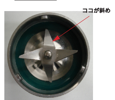
回転方向（時計回り）に対して 刃が斜め
